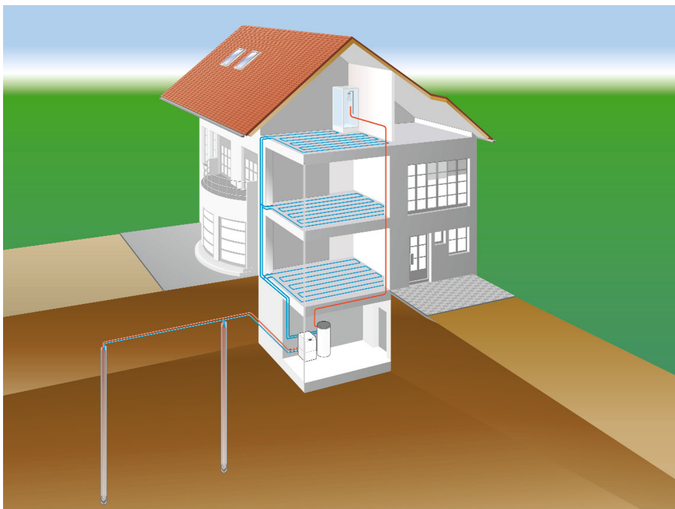
Exemple d'une pompe à chaleur sol/eau en refroidissement passif
