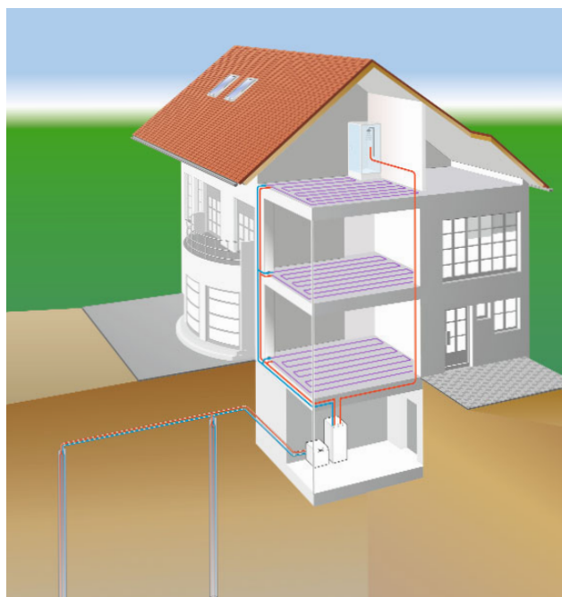
Sondes géothermiques
