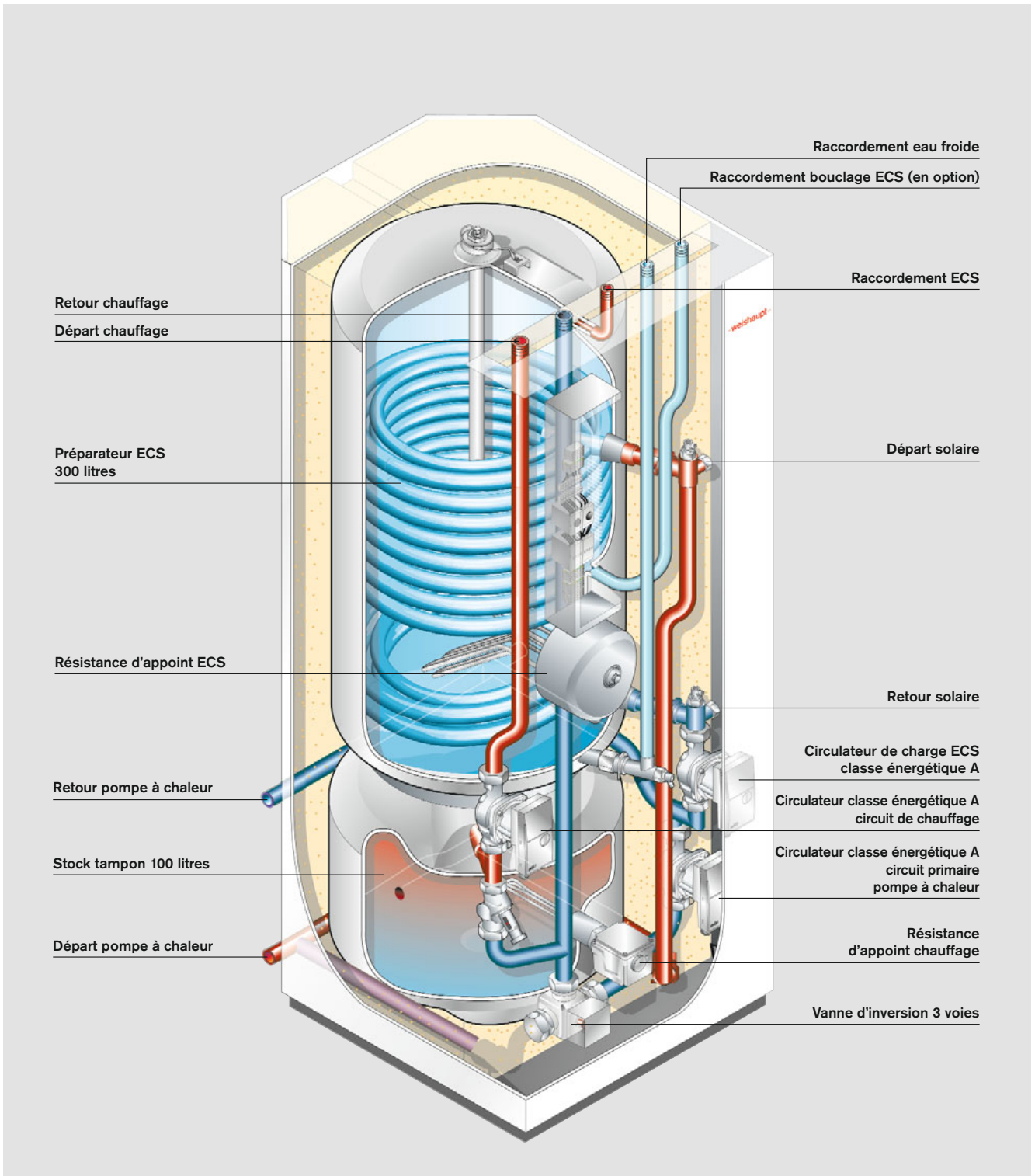
Préparateur multifonction Weishaupt WKS 300/100 LE/Unit-E/Block
